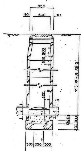
橫断面図
