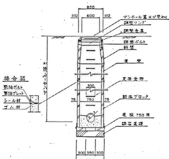
橫断面图
