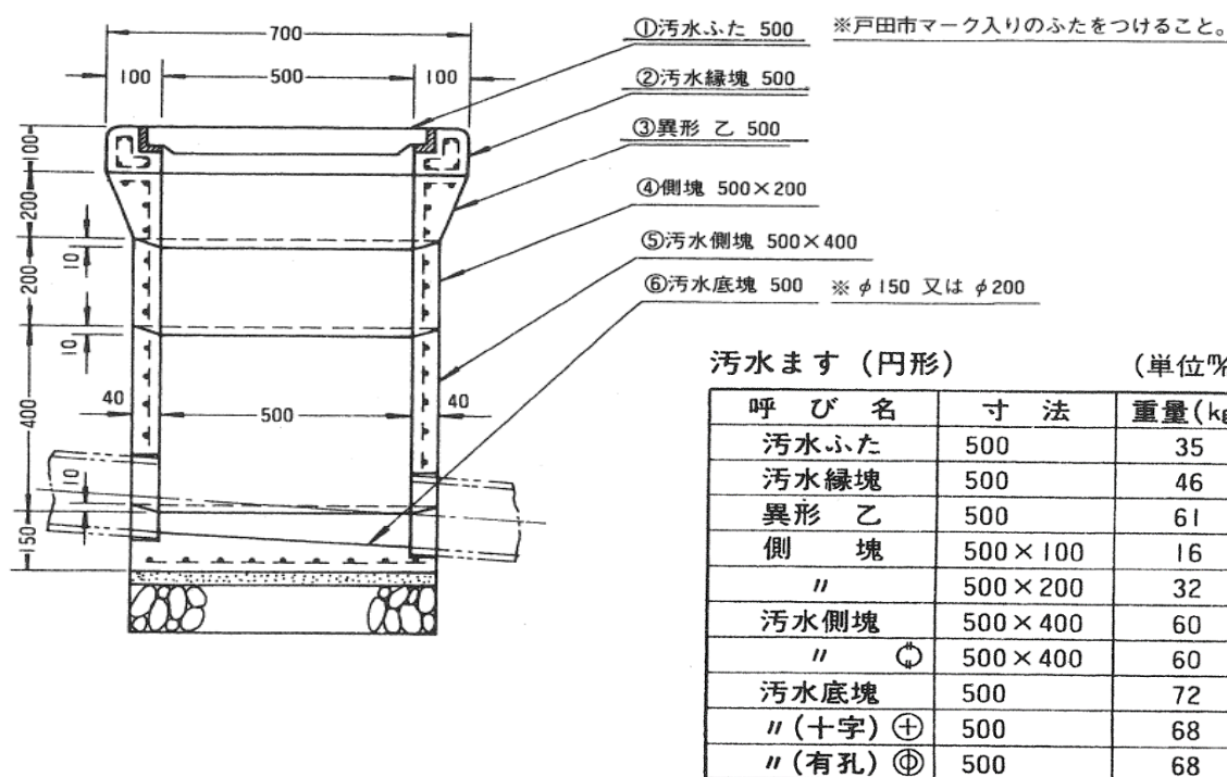
汚水ます（円形）500用
