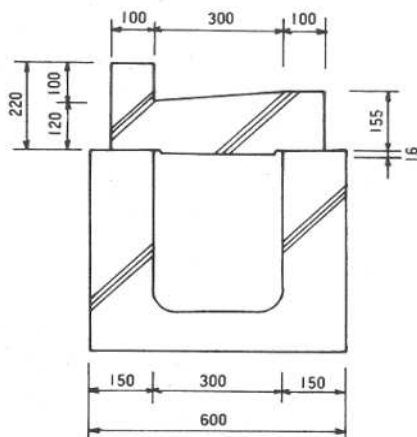
図 - 8 特殊 LU 型側溝
