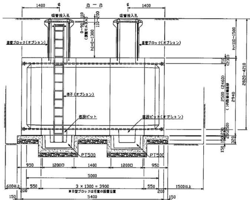
側面図
