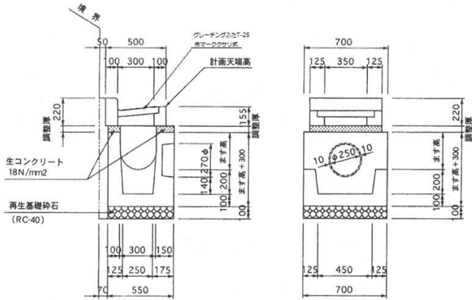
● 図-11 集水ます (B) (S = 1:20)
