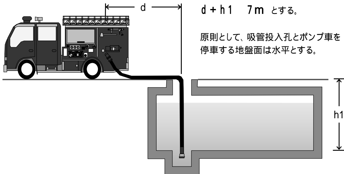
防火水槽の設置場所参考図（第5図）
