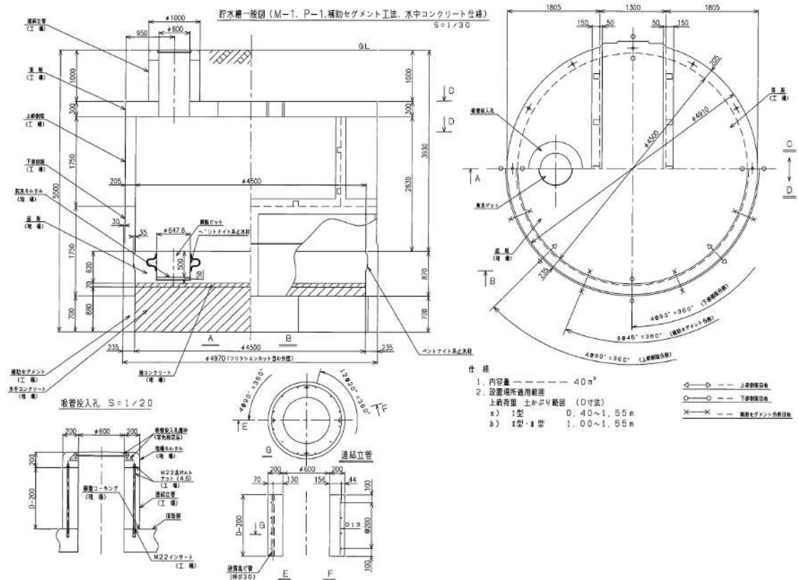
二次製品防火水槽（縦円筒型）参考図（第3図）
