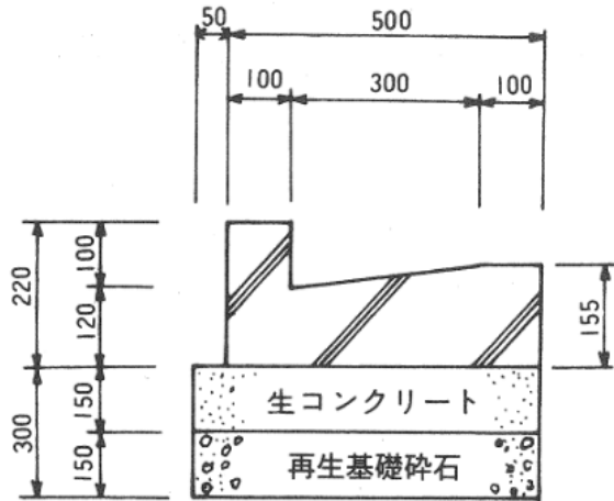
●図-2 特殊L型側溝 (単位mm)
