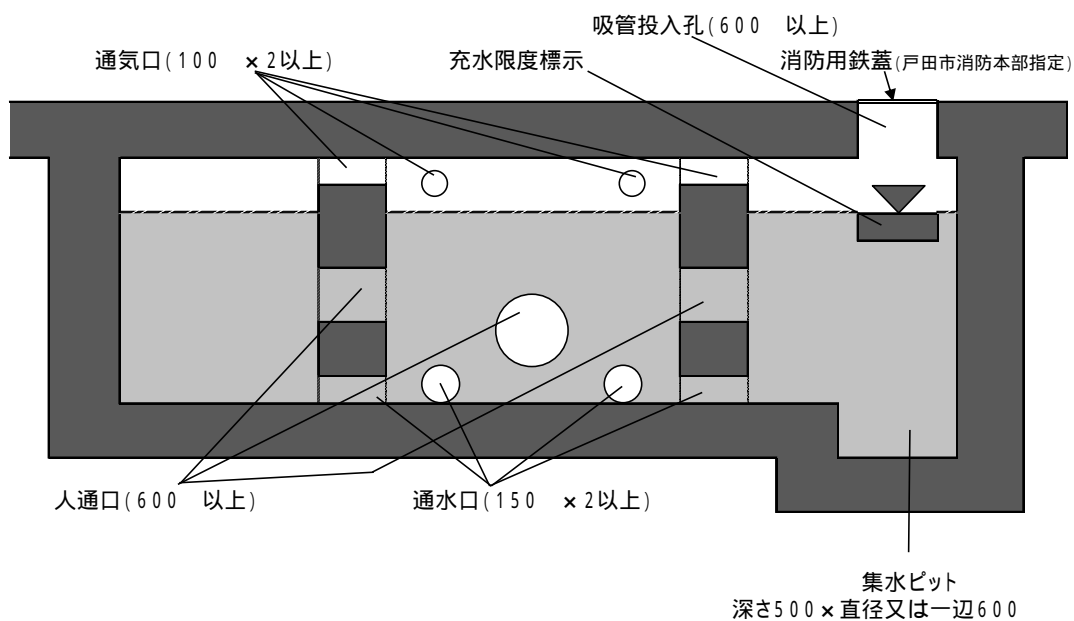
地中ばり防火水槽参考図（第4図）
