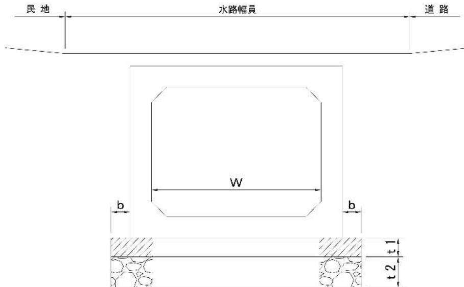
図-1 出入口（ボックスカルバート）標準断面図（参考図）
