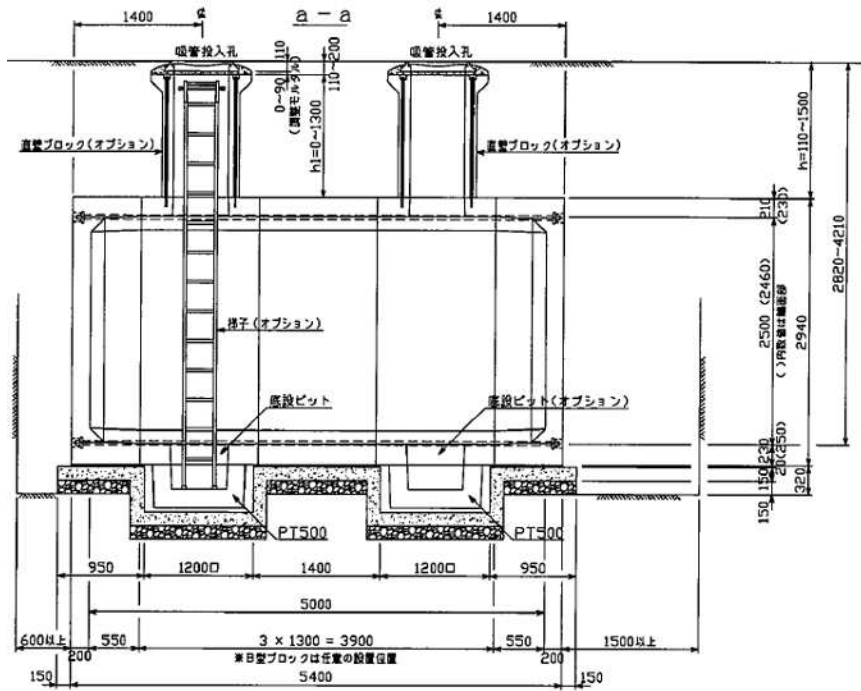
二次製品防火水槽（縦円筒型）参考図（第3図）
