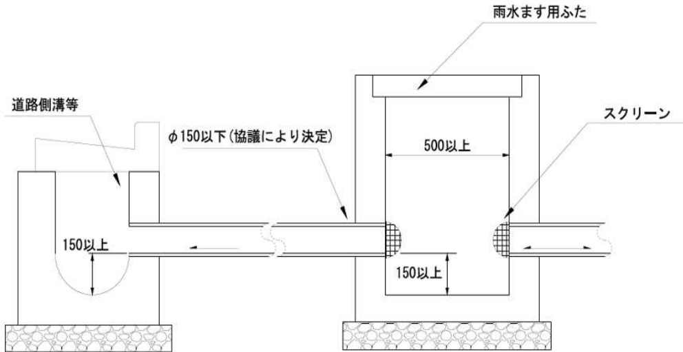
雨水ます及び排水管 (単位mm)
