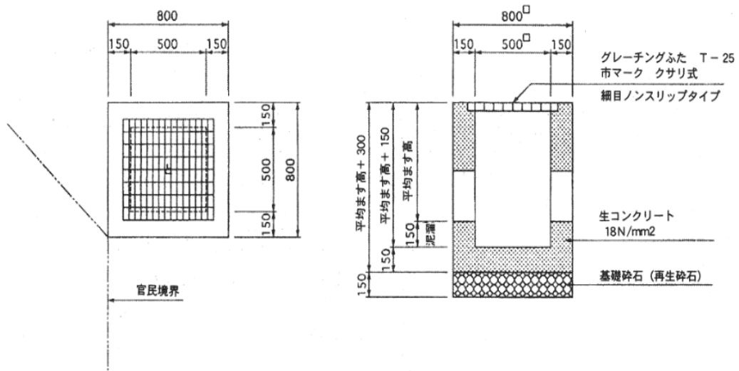
● 図-11 集水ます (B) (S = 1:20)
