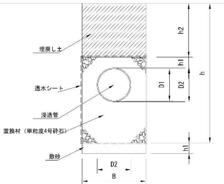
図-2 浸透施設標準構造図（参考図）
