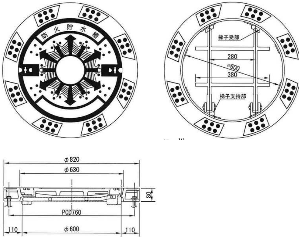
防火水槽蓋参考図（第6図）
