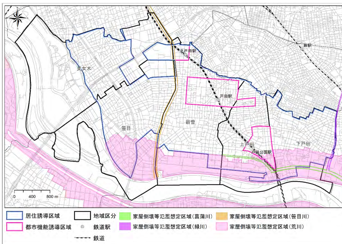
図 3-12 家屋倒壊等氾濫想定区域図
