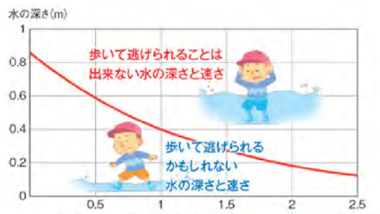
図3-9 水の中を歩くことができる範囲
