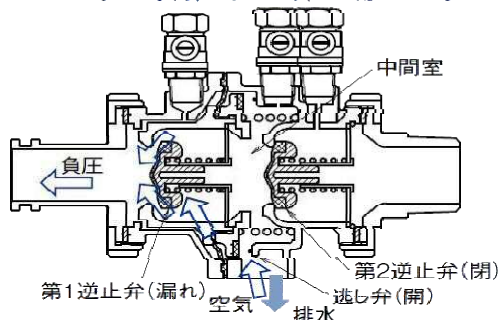
逆サイフォン時、第1逆止弁が漏れた時
