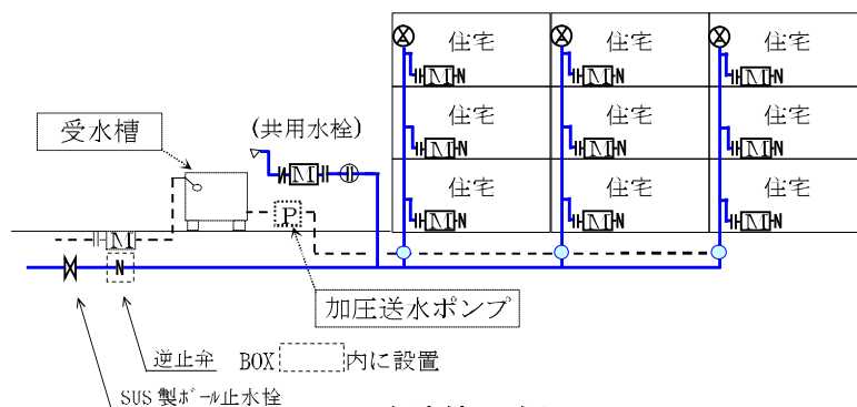
改造施工例一 2
