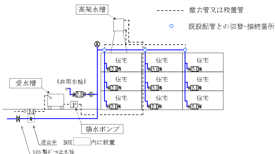
改造施工例一 1
