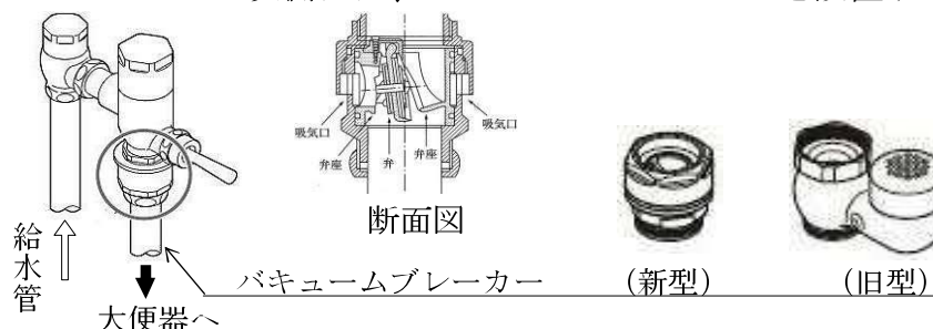
大便器洗浄弁のバキュームブレイカー
