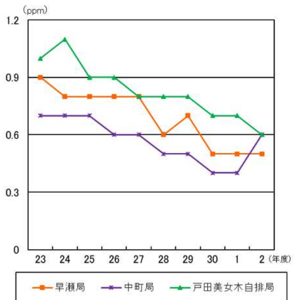
図 4-2-9 一酸化炭素 2%除外値経年変化
