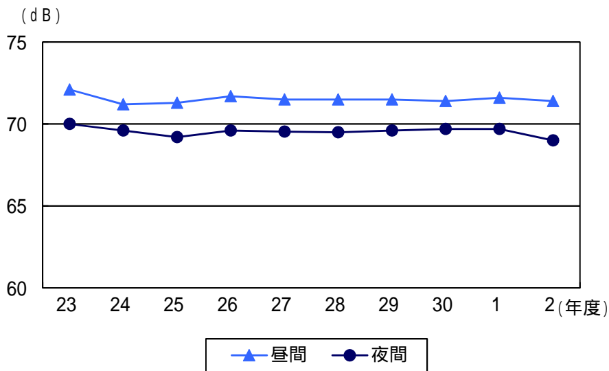
図 4-4-6 美笹局騒音経年変化
