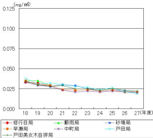
図 3-2-10 浮遊粒子状物質年平均値経年変化
